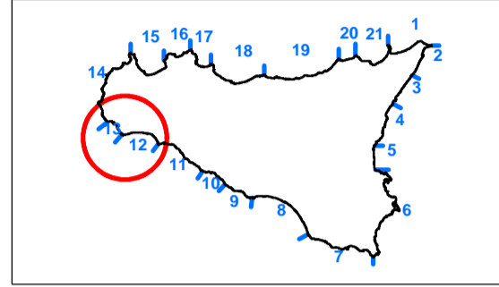
Carta della tipologia costiera e dell'evoluzione delle linee di riva N°3 Scala 1:5.000
