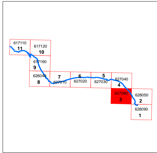
Carta della tipologia costiera e dell'evoluzione delle linee di riva N°3 Scala 1:5.000
